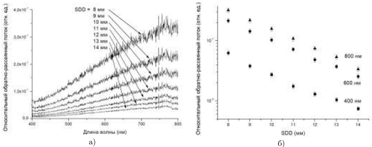
Рис. 4: а) Экспериментально измеренные спектры относительного обратного-рассеянного потока F для образца толщиной 10 мм при различных значениях расстояний источник-детектор (SDD); б) зависимости F от SDD для трех длин волн (400, 600 и 800 нм)
